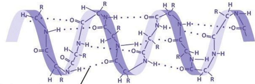
α helix
