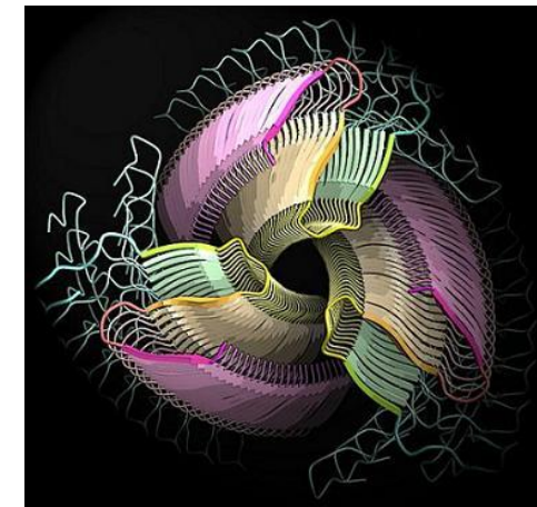
Амилоидные фибриллы
