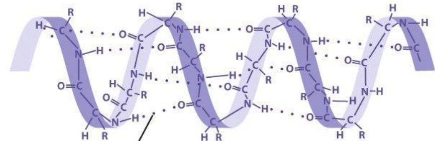
α helix
