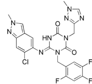
5 S-217622
