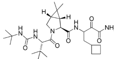
11 Boceprevir
