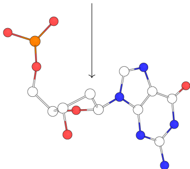
B-DNA C2'-endo
