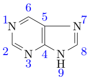
Пурин
