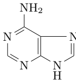
Аденин
